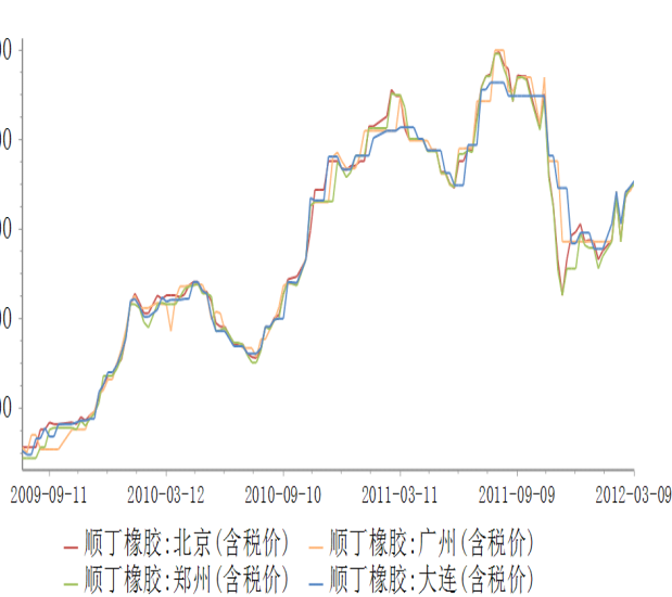
图 表 8: 顺丁橡胶 (单位: 元/吨)
