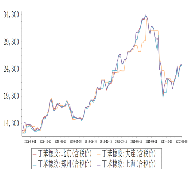
图 表 7: 丁苯橡胶 (单位: 元/吨)
