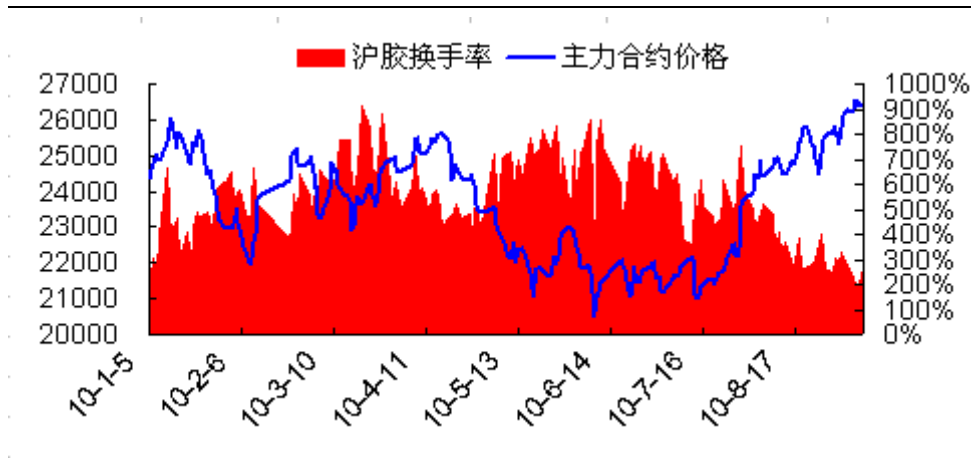
图3：沪胶换手率
