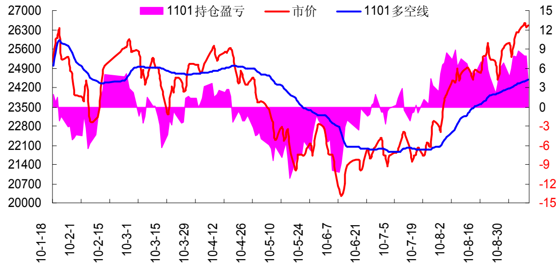
图1：1101多空线
